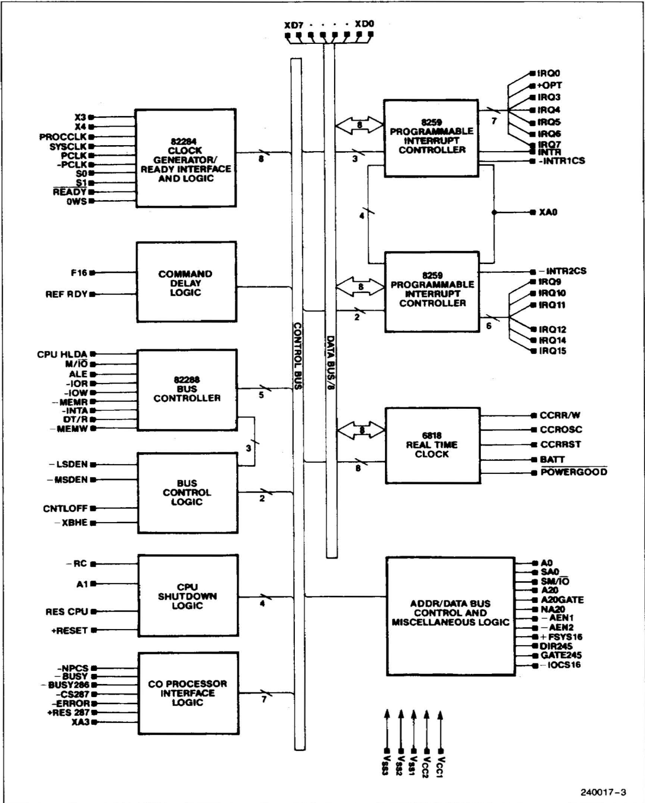
82230—Block Diagram
