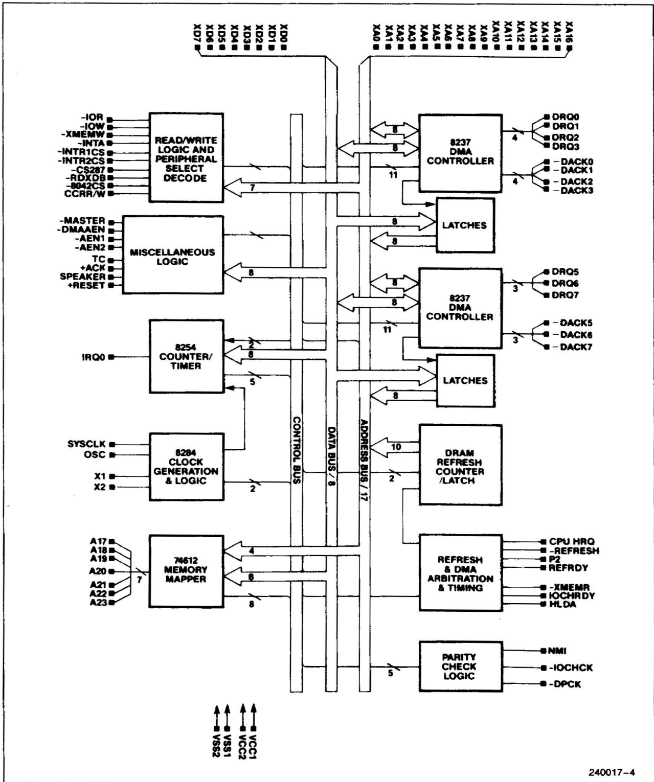
82231—Block Diagram
